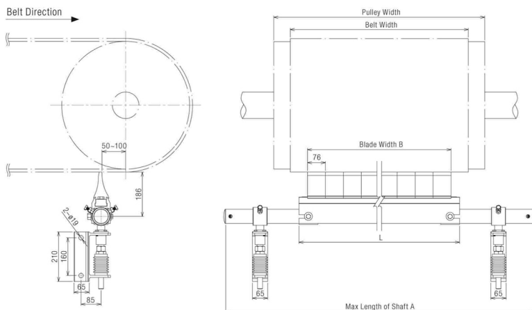
Tungsten Carbide Blade – SBC2
